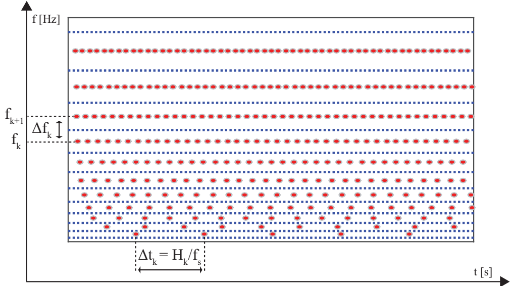
(b) CQT
